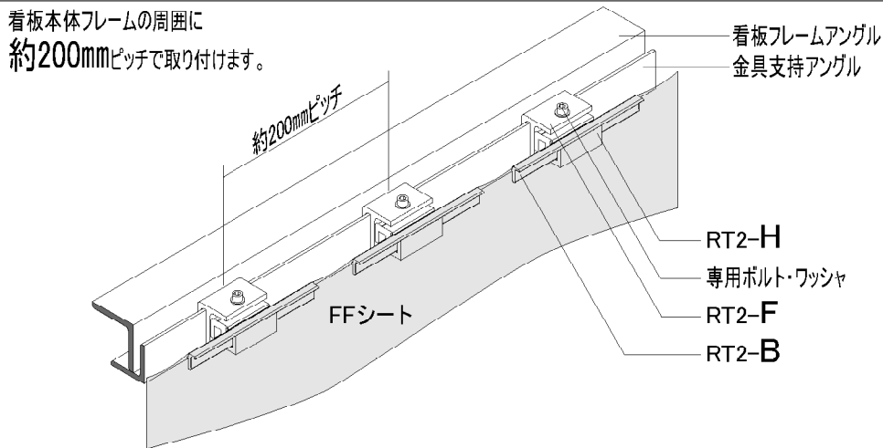
専用ボルト・ワッシャ (M6 x 40mm SUS)
